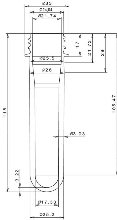
A-A View/Görünüm
